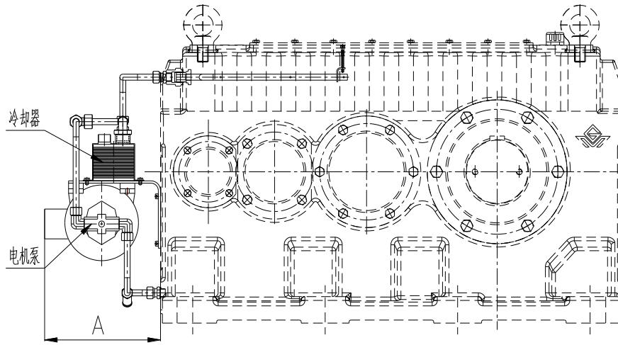
附表 D1 强制润滑尺寸
